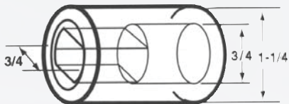
7DD - 3/4" DD x 3/4" smooth
